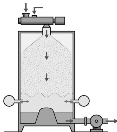
図8 漂白タワー
