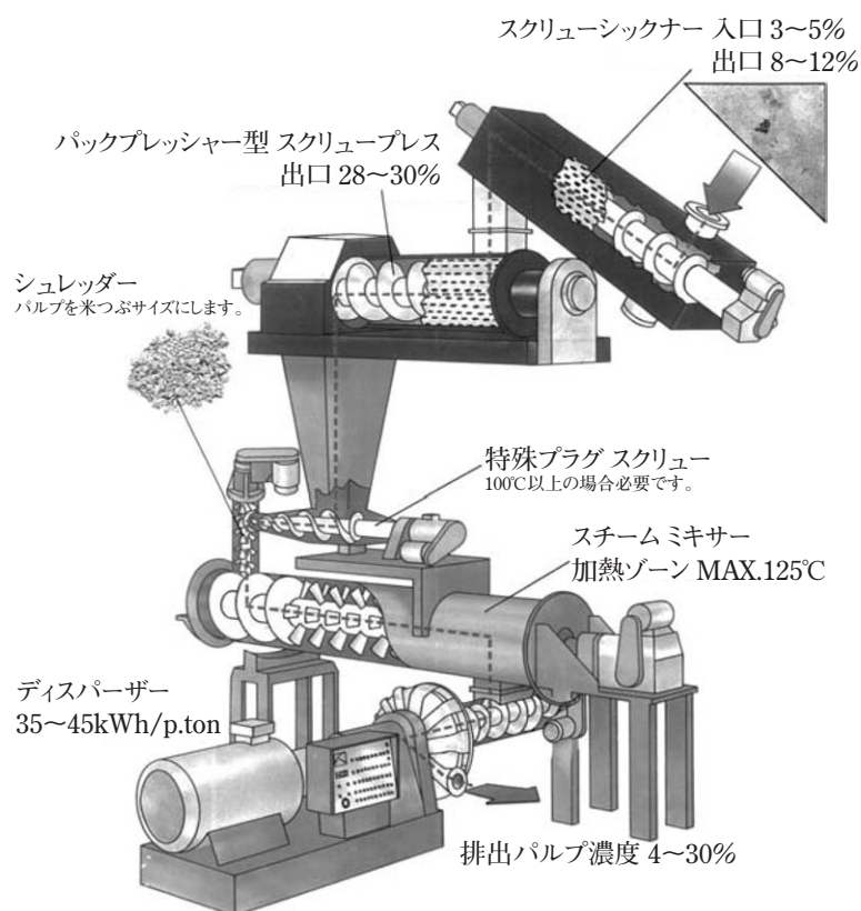
図 21 ホットディスパーザー設備
